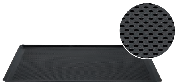
Teglia gastronorm 1/1 microforata (ø foro 2 mm) in lega 3003 rivestita con antiaderente
